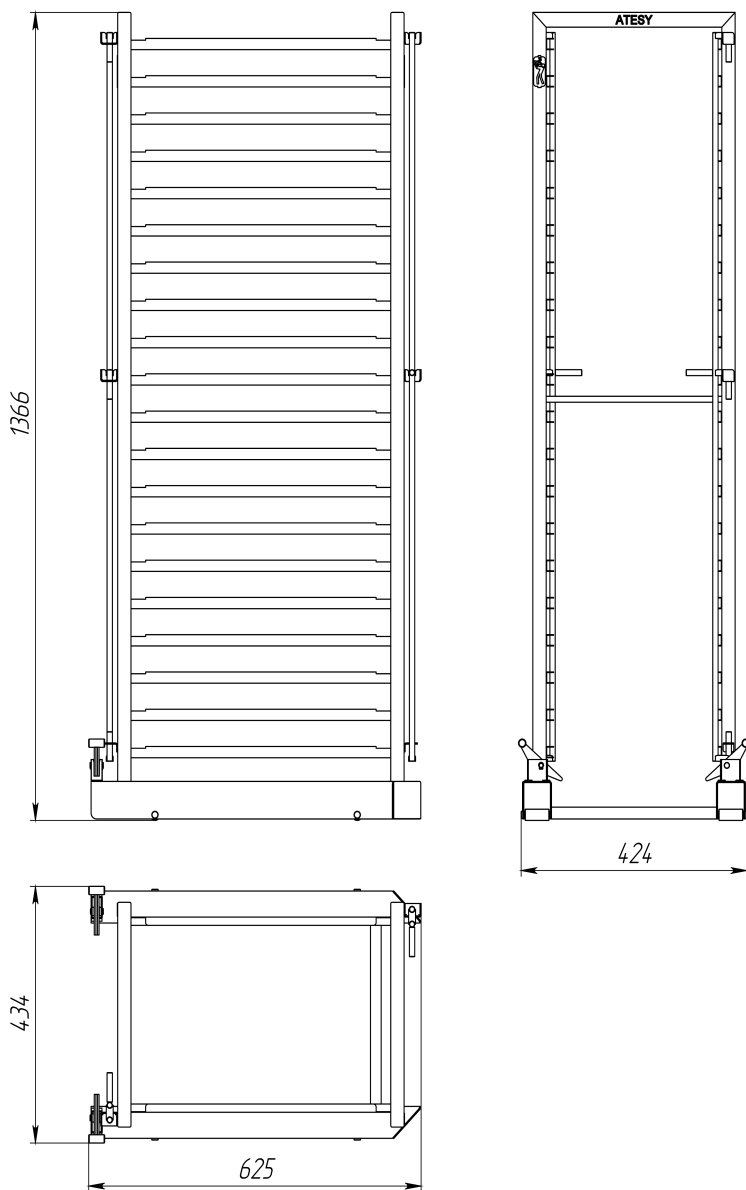
Рис. 1 Общий вид.
