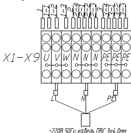
Рис.2 Подключение к однофазной сети
