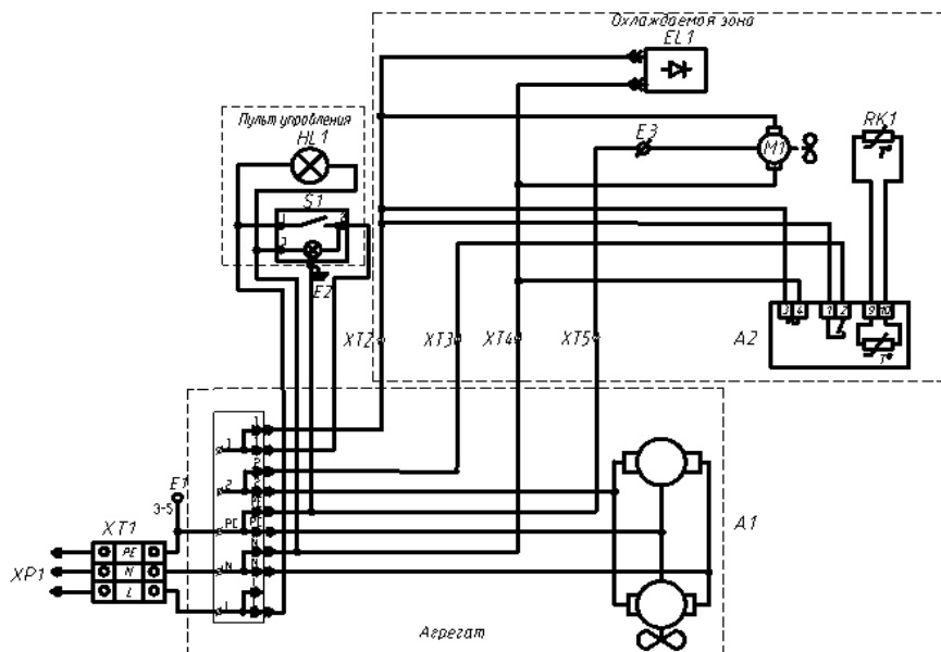
Схема электрическая принципиальная.
